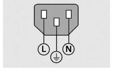
Güç kablosu
