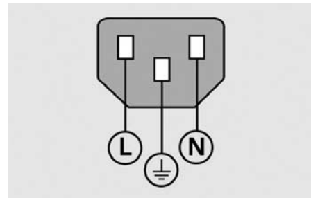
Καλώδιο τροφοδοσίας
