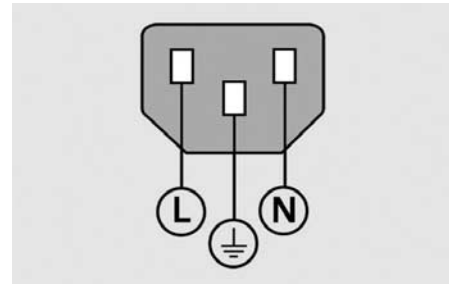
Tápkábel
