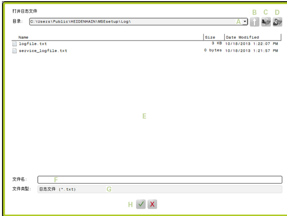
文件对话框
