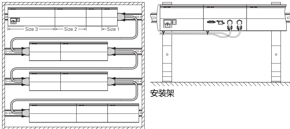
19"机柜
