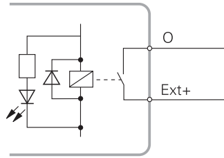
外部电源
