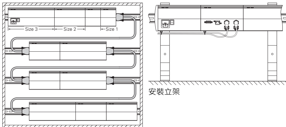
19" 安裝機櫃
