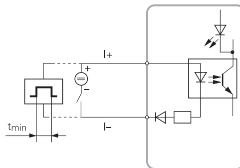
外部電源
