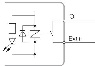
外部電源
