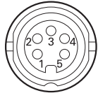
Разъем датчика
