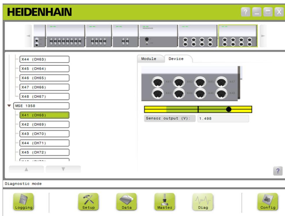
Окно диагностики датчиков LVDT
