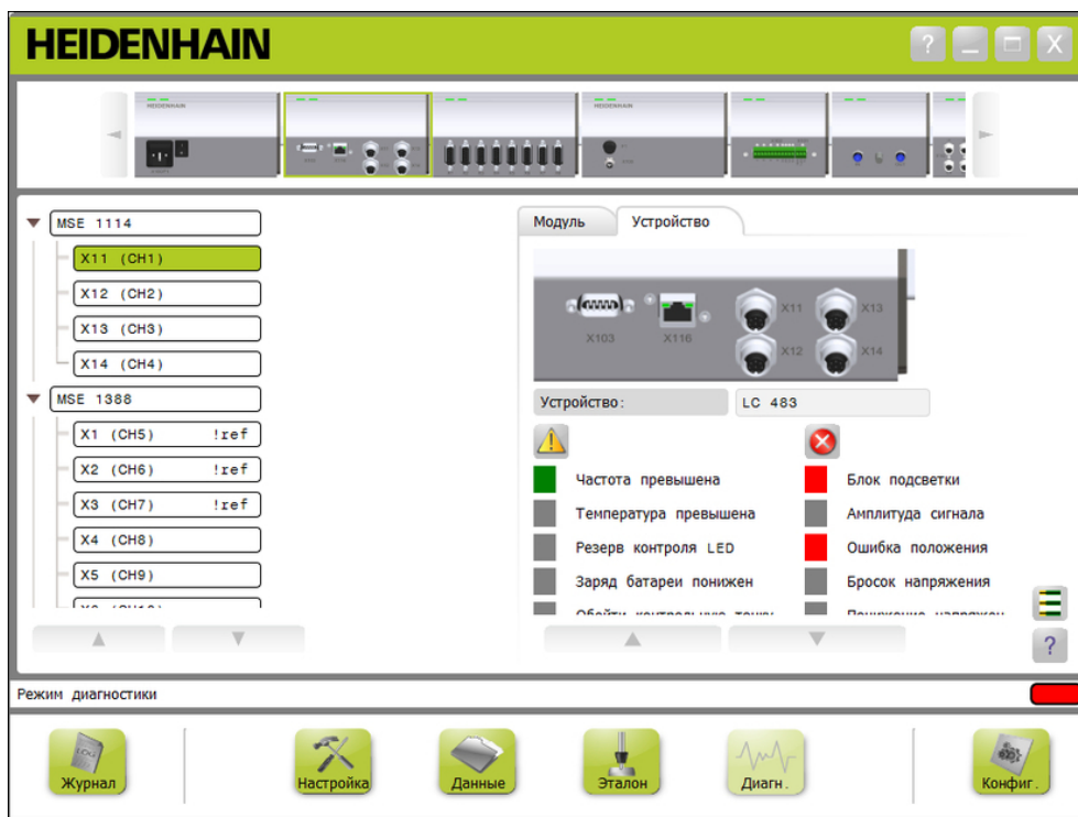
Окно предупреждений и ошибок датчиков с интерфейсом EnDat
