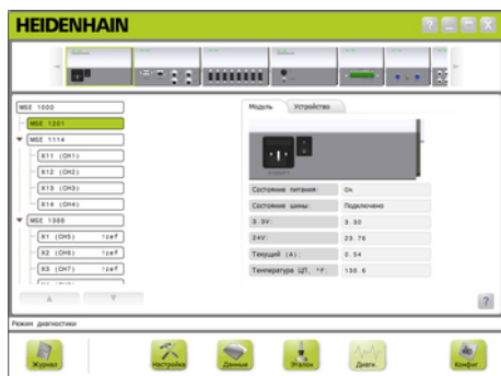
Окно диагностики модуля питания
