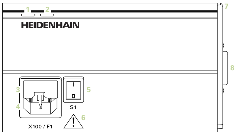
Передняя панель MSE 1201 ID 747501-02
