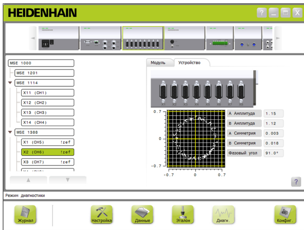
Окно диагностики датчика 1 V PP
