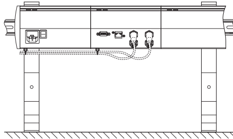
Montaj standı
