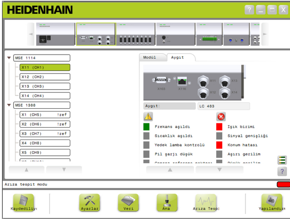
EnDat uyarıları ve hataları ekranı
