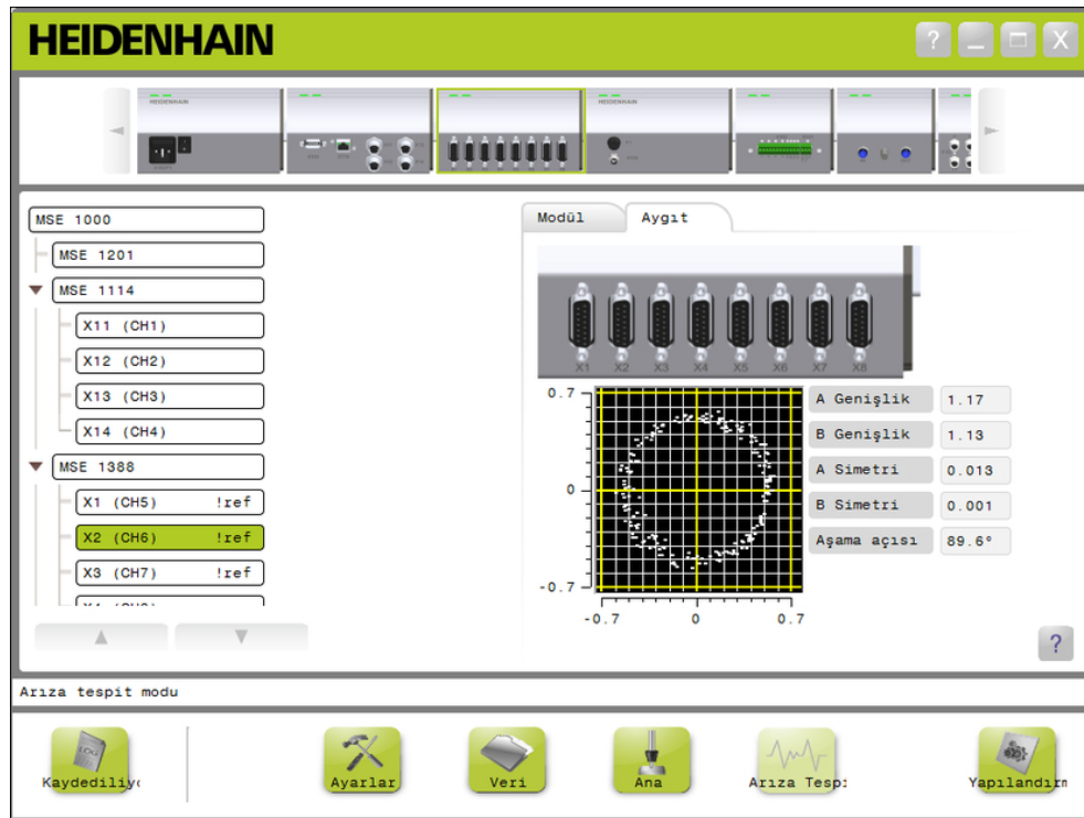
1 V PP arıza tespit ekranı
