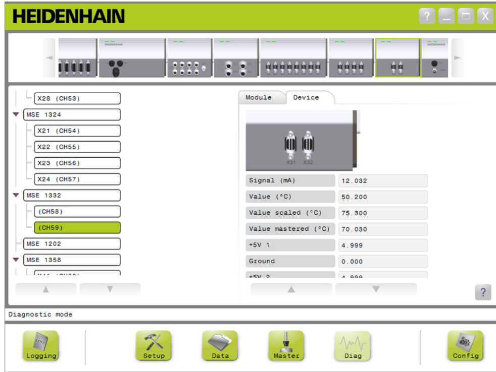
Analog arıza tespit ekranı
