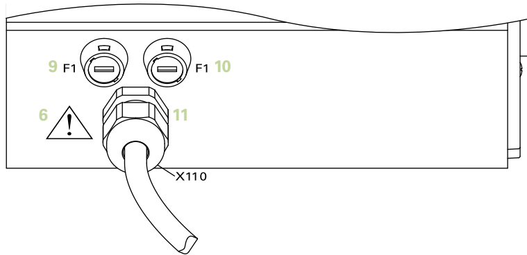
MSE 1202 전면 ID 747502-0x
