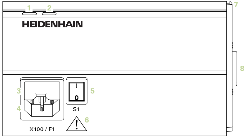
MSE 1201 전면 ID 747501-02
