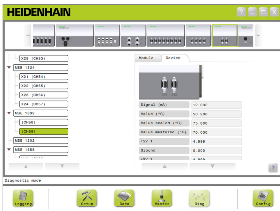
アナログ診断画面
