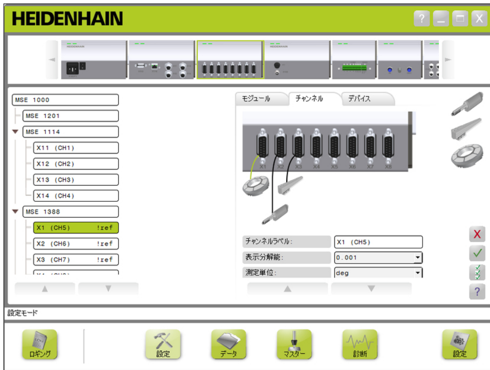
チャンネル設定タブ
