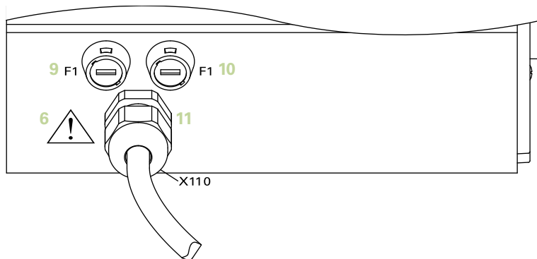
MSE 1202の前面 ID 747502-0x
