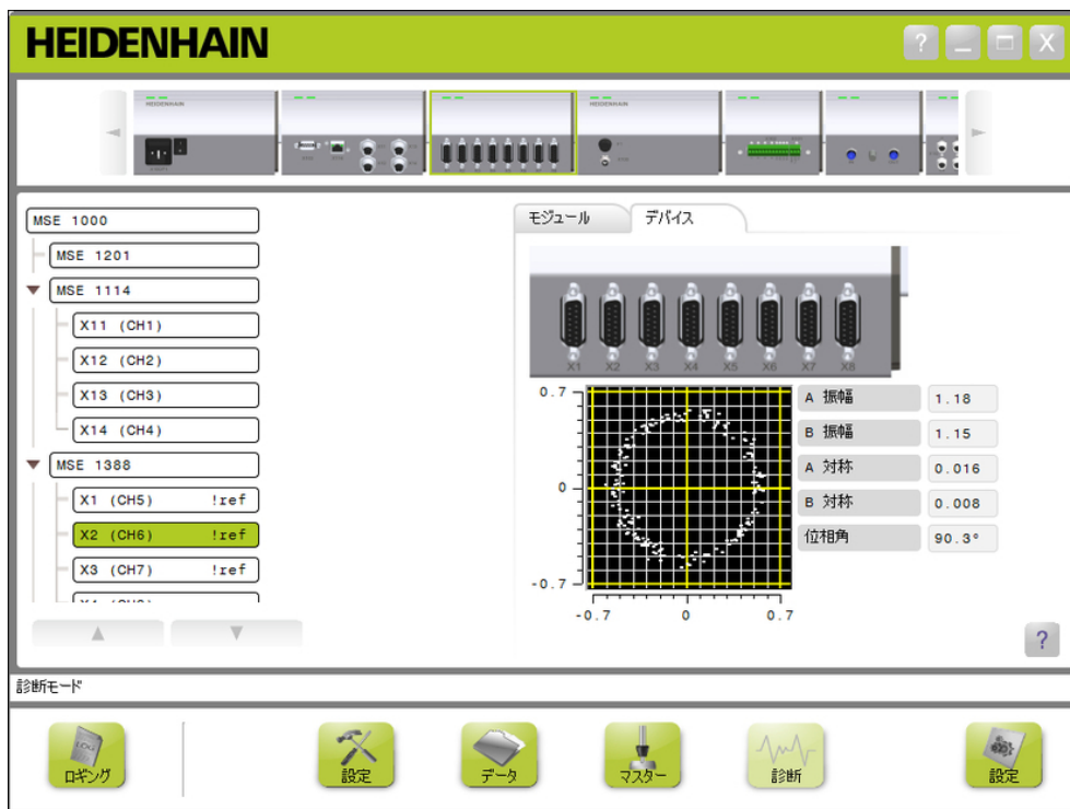
1 V pp 診断画面
