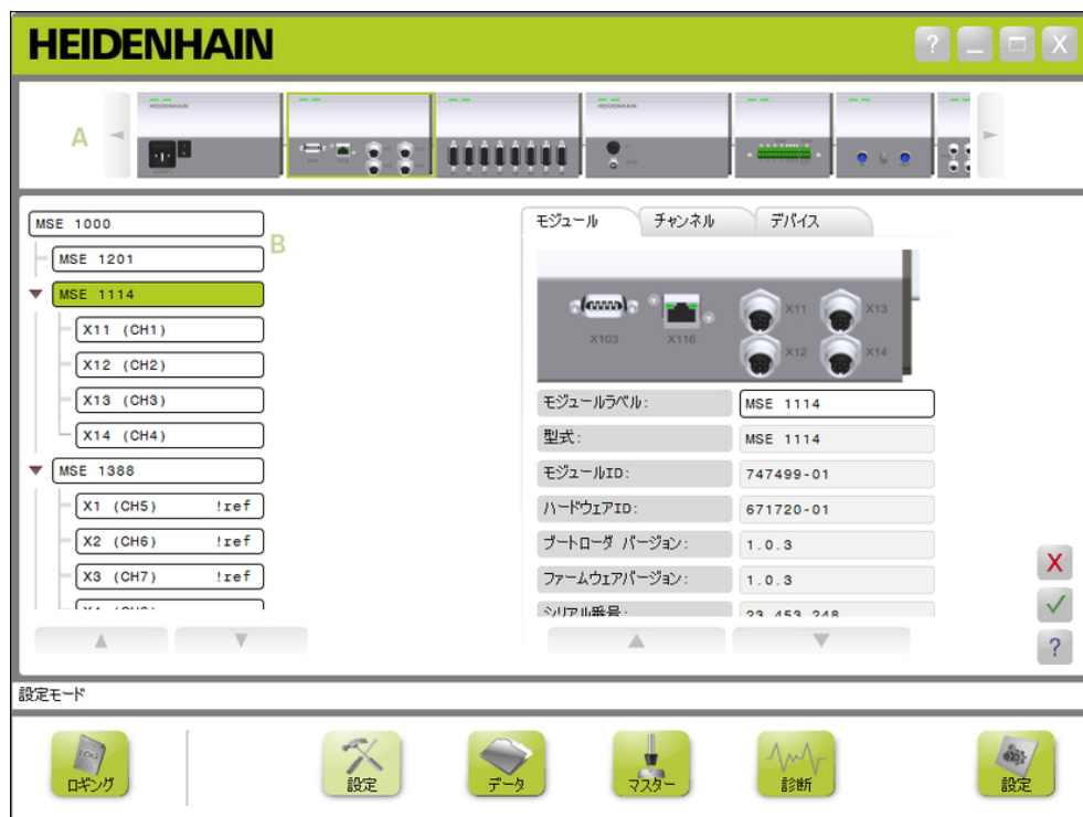
アプリケーションウィンドウのモジュールビューおよびツリービュー
