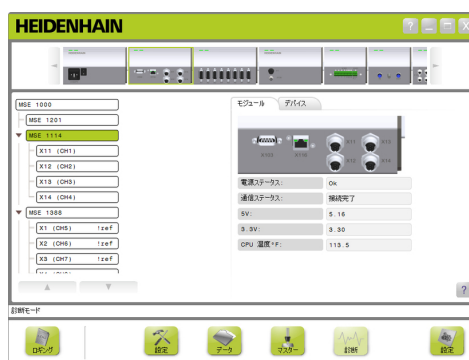
電源モジュール以外の診断画面
