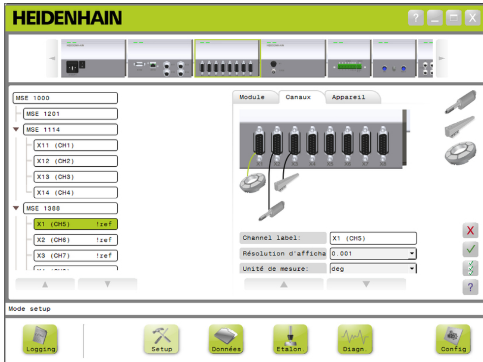
Onglet de configuration "Canal"
