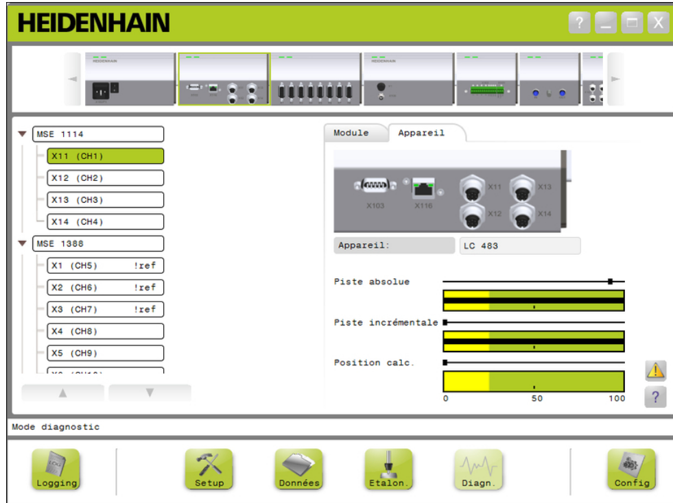
Ecran Réserves fonctionnelles
