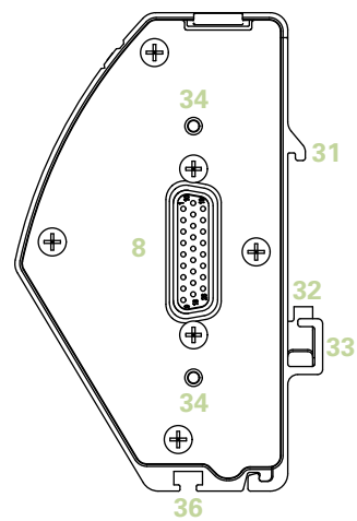
Côté droit
