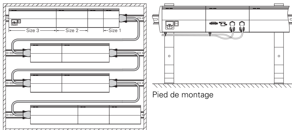
Armoire de montage 19 pouces
