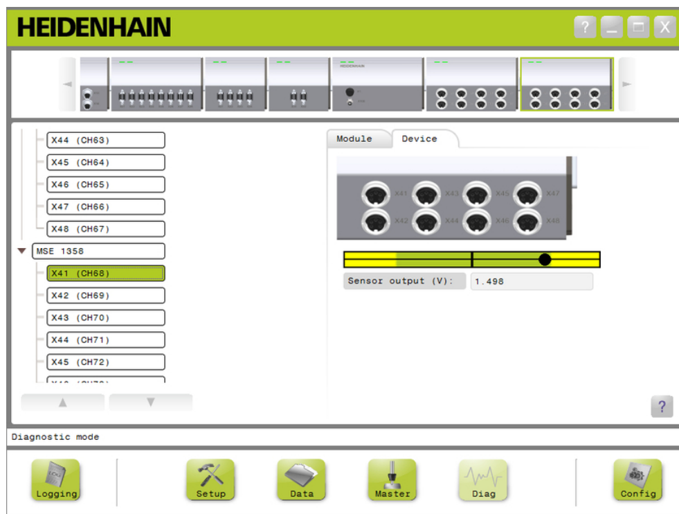
Ecran Diagnostic des palpeurs LVDT
