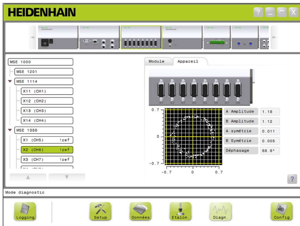
Ecran de diagnostic 1 V CC
