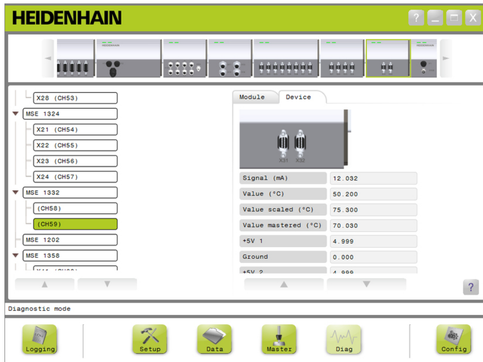
Ecran de diagnostic analogique
