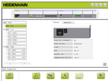
Ecran de diagnostic des modules d'alimentation
